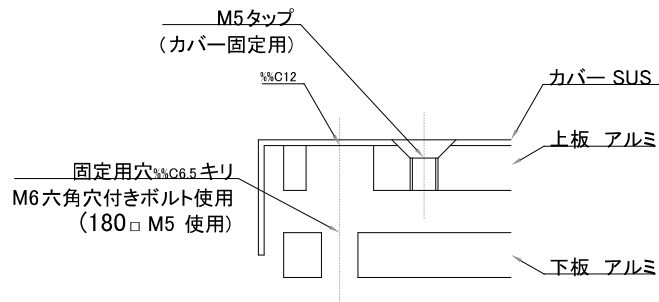
A-A'断面
